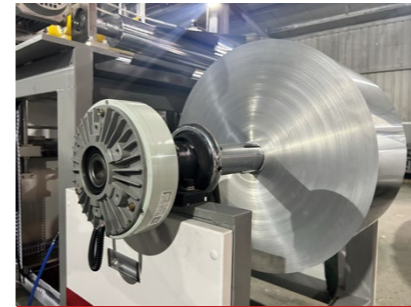
放料张力控制系统 Unwinding tension control system
